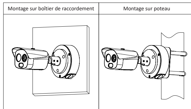
PFA152-E Support de montage sur mât
