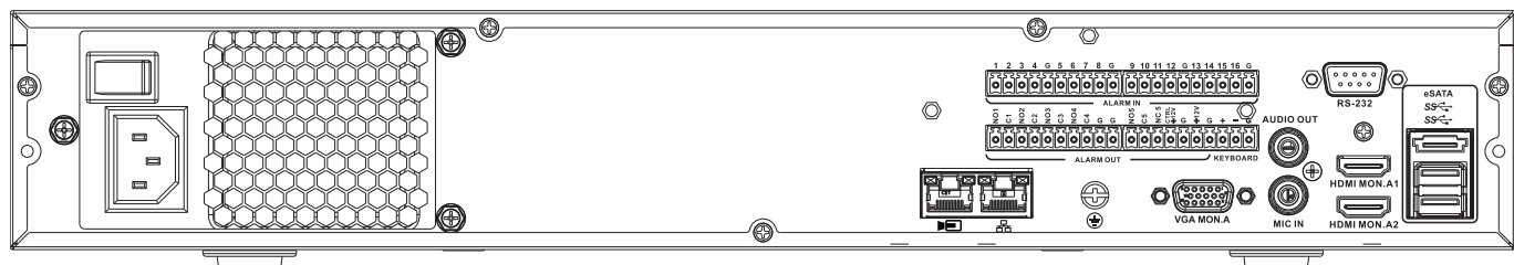
Achterpaneel DIVAR network 5000 (geen PoE)
